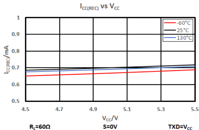
图 7-2 隐性状态电流
