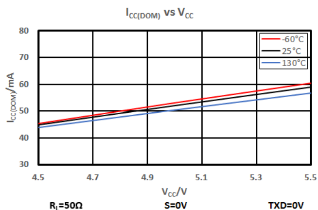
图 7-3 50Ω 负载下显性状态电流
