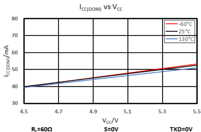
图 7-4 60Ω 负载下显性状态电流
