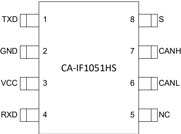
图 6-1 CA-IF1051HS 引脚图
