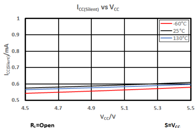
图 7-1 静默态电流
