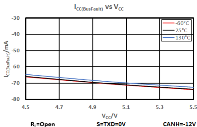
图 7-5 总线故障电流
